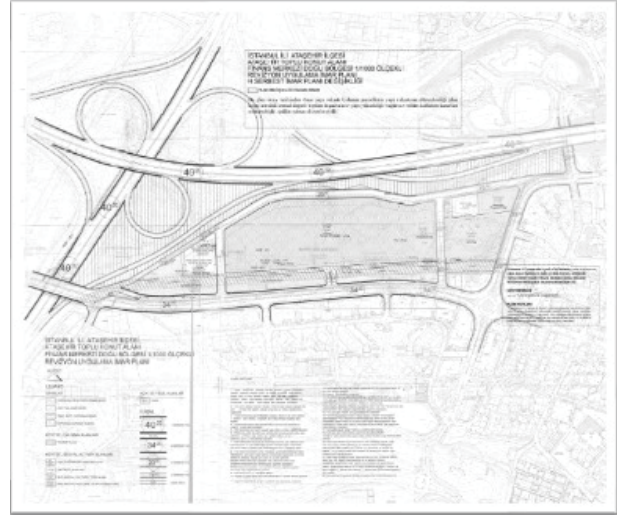
İstanbul İli, Ataşehir İlçesi, Ataşehir Toplu Konut Alanı Finans Merkezi Doğu Bölgesi 1/1000 Ölçekli Revizyon Uygulama İmar Planı H Serbest İmar Planı Değişikliği
